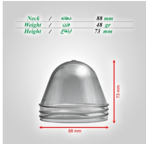
پریفورم جار پت دهانه ۸۸ نرمال نک ۴۸ گرم
